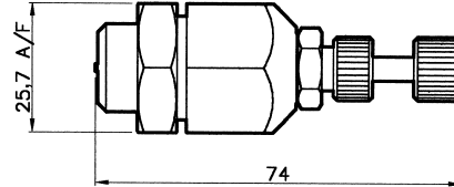
1/8" AL - A (Manual metering needle) Durchfluss Regulierung per Hand
