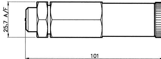
1/8" AL Variante 5F
